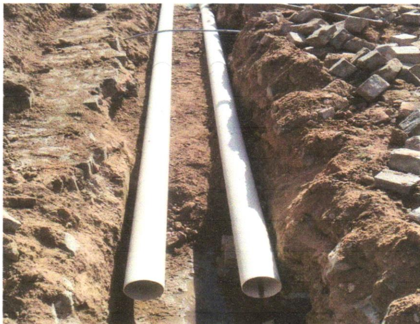
FOTO 04 - ESCAVAÇÃO MANUAL DE VALA COM PROFUNDIDADE MENOR OU IGUAL A 1,30 M
